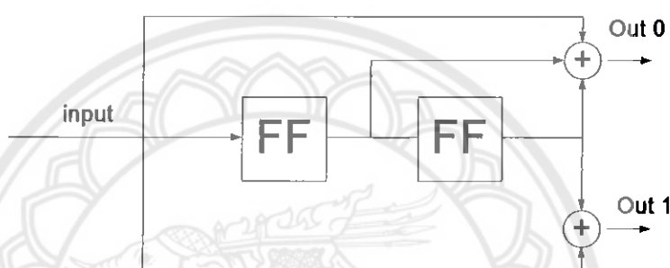
รูปที่ 4.3 การเข้ารหัสแบบ Convolutional code ที่ K=3 Rate 1/2
