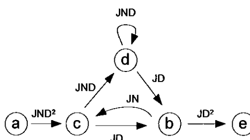
รูปที่ 4.4 State diagram Rate 1/2
