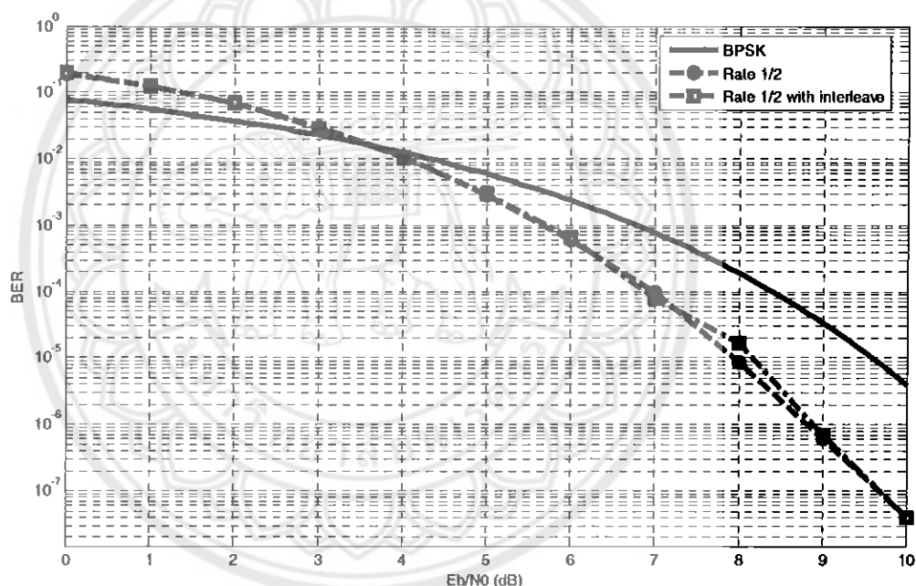
รูปที่ 4.8 แสดงการเปรียบเทียบ BER Convolutional Code (Hard-decision) ระหว่างที่มีการใช้
