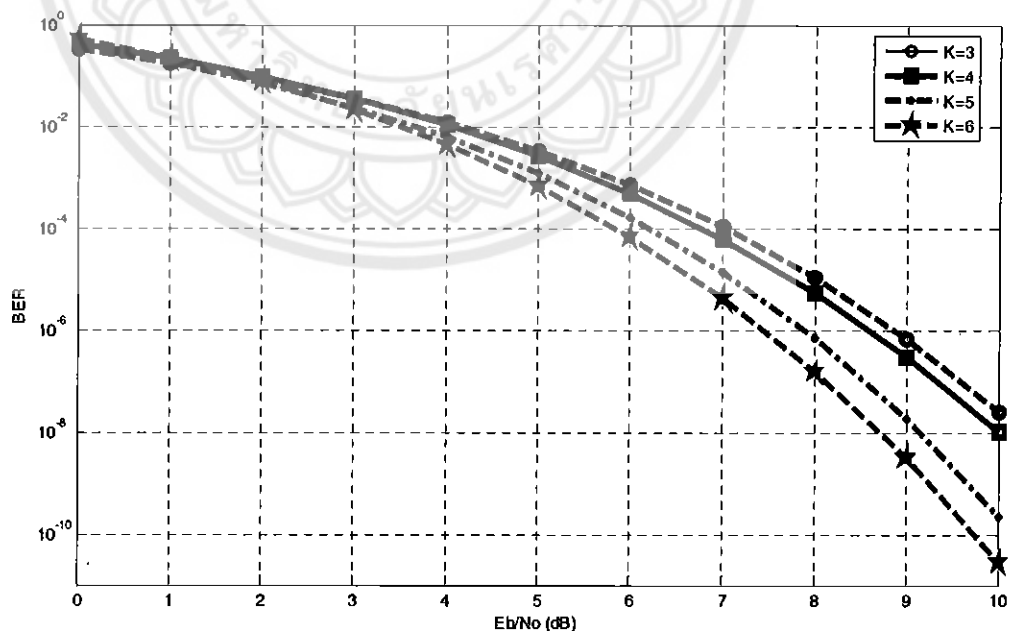
รูปที่ 4.1 กราฟ BER Convolutional Code R=1/2 โดยใช้วิธีแบบ Hard-decision
