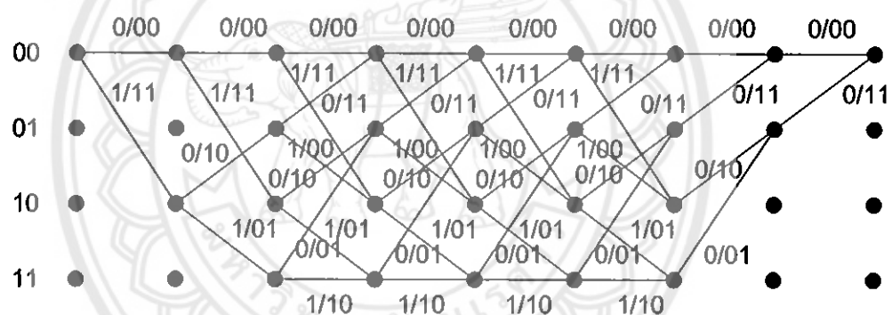
รูปที่ 2.6 แสดงการนำค่าที่ได้จาก State diagram มาสร้างแผนภาพเทรลิส
