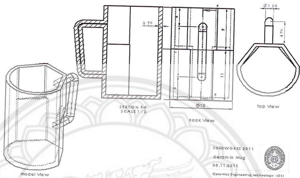
ภาพแบบเขียนแบบ (Drawing) แก้วม็อค
