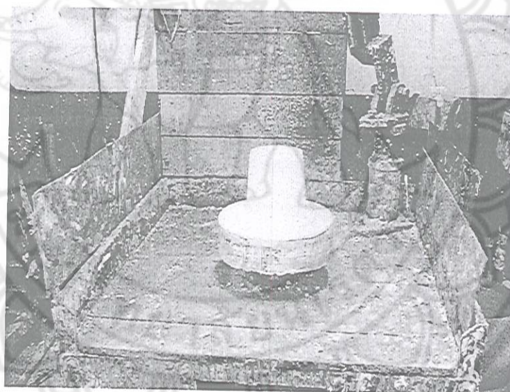
ภาพการเทพิมพ์ต้นแบบเป็นทรงกระบอก
