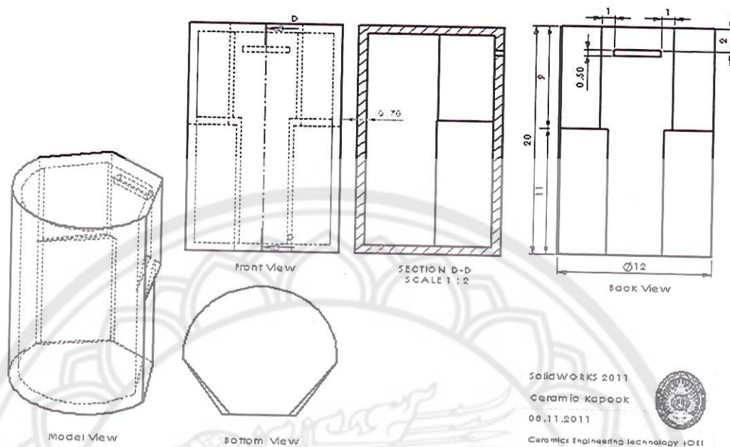
ภาพแบบเขียนแบบ (Drawing) กระปุกออมสิน
